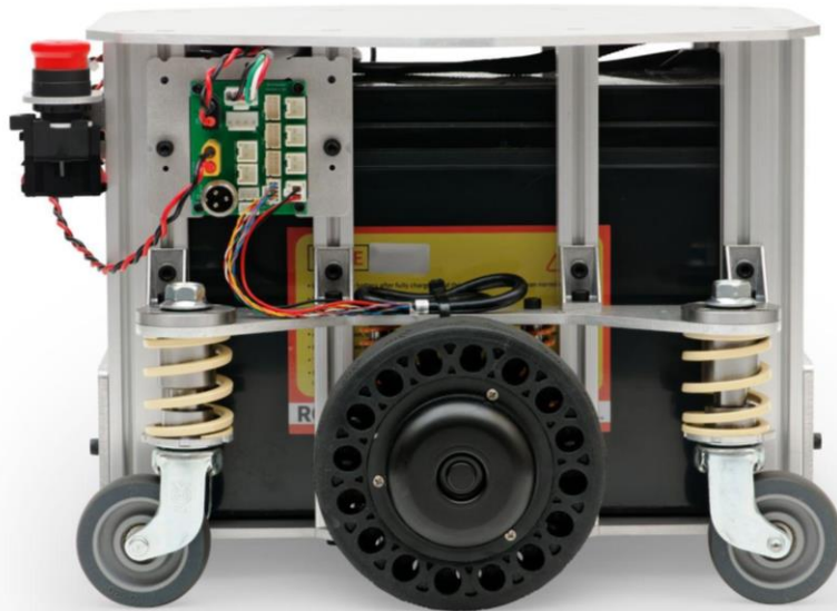
駆動輪を車体の前後方向に対して中央に配置
