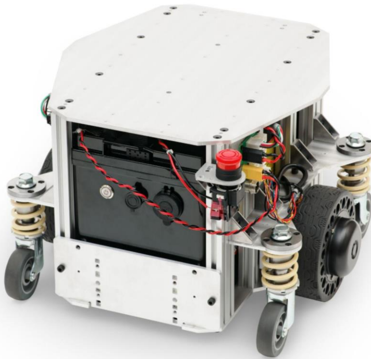
メガローバーS40A-LB
